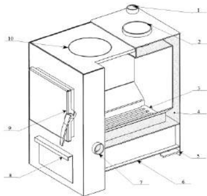
Рис. 1 Схема устройства котла.
