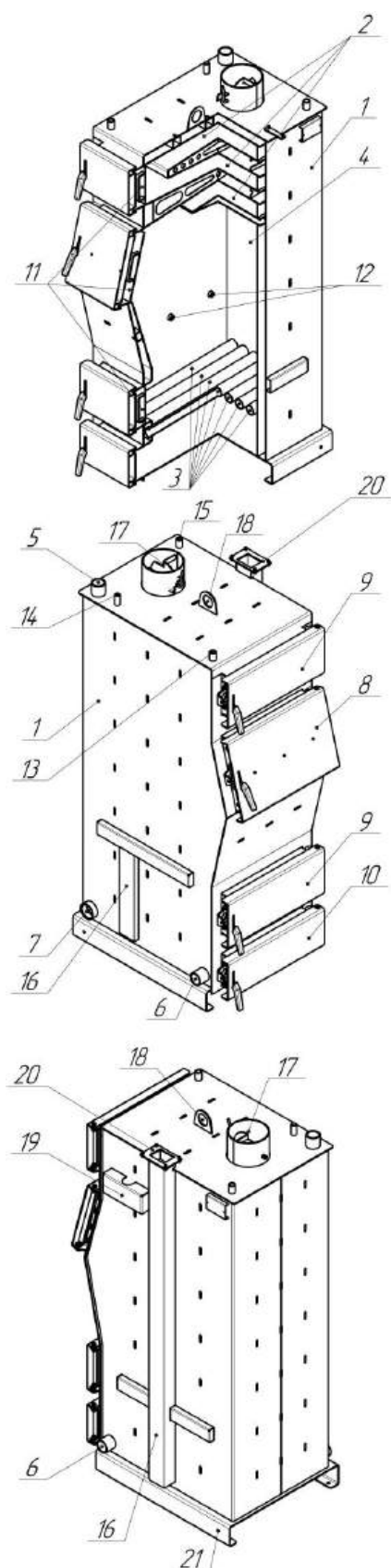
Рис. 5 Схема устройства отопительного кола HUNTEL «SARMAT».
