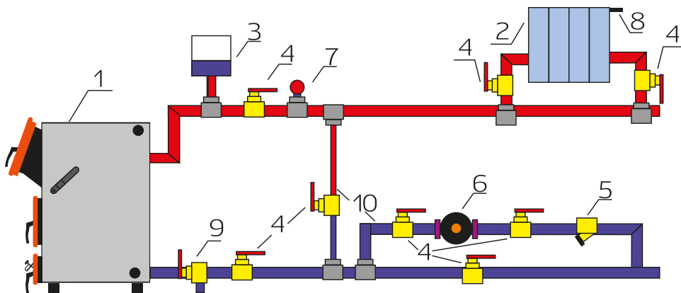
Подключение котла к одноконтурной открытой системе с принудительной циркуляцией теплоносителя:
