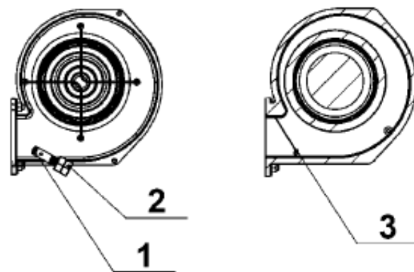
Рис. 7 Установка заслонки вентилятора (положение закрыто)
