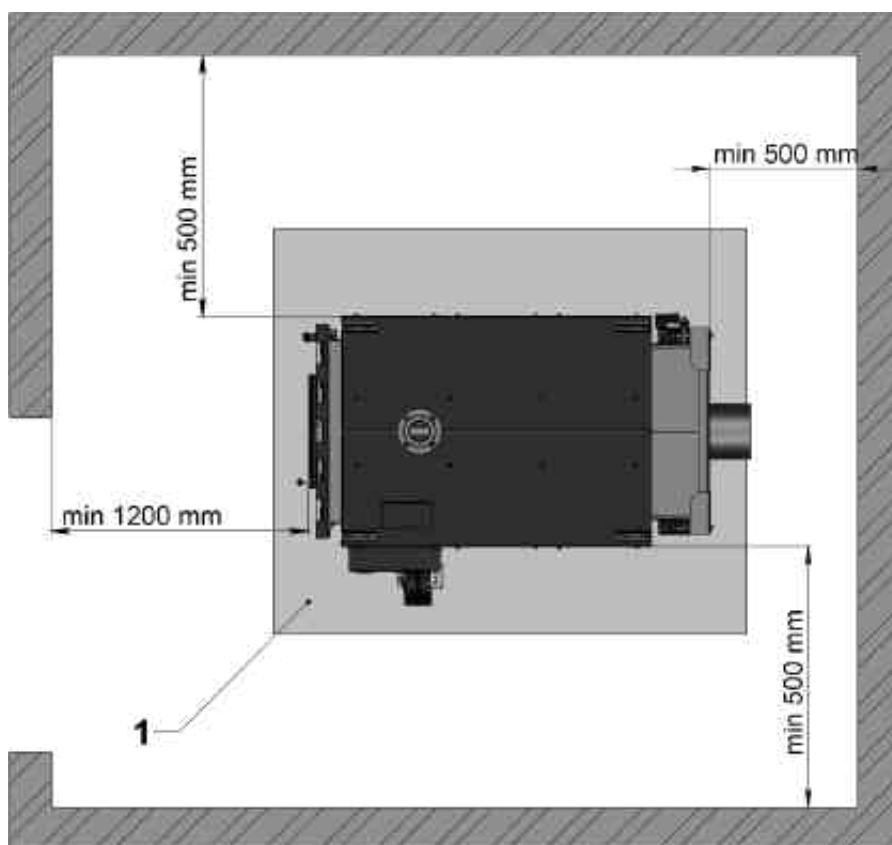
Рис. 4 Установка котла
