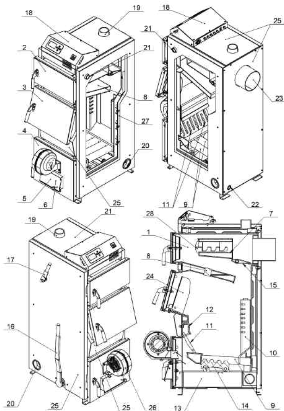
Рис. 2 Устройство котла
