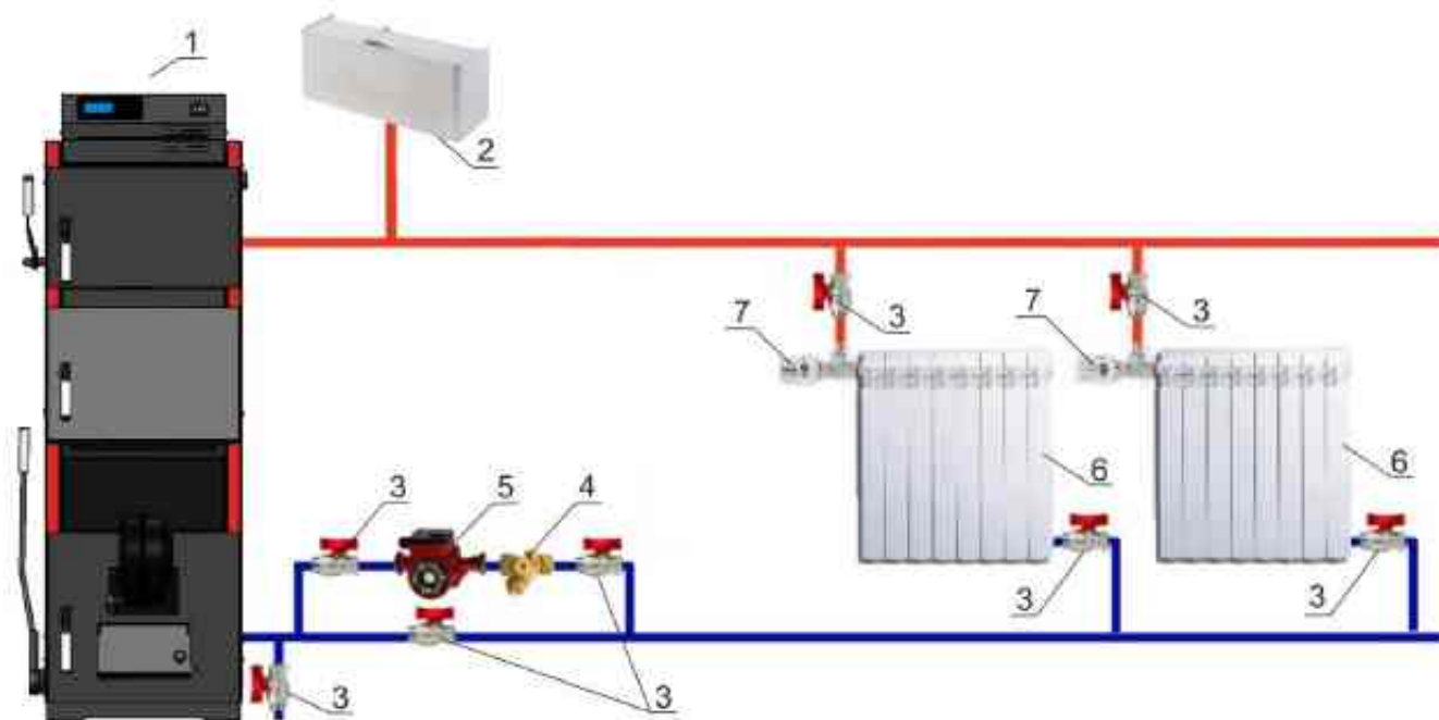
Рис. 5 Схема подключения котла к открытой системе с принудительной циркуляцией теплоносителя 1
