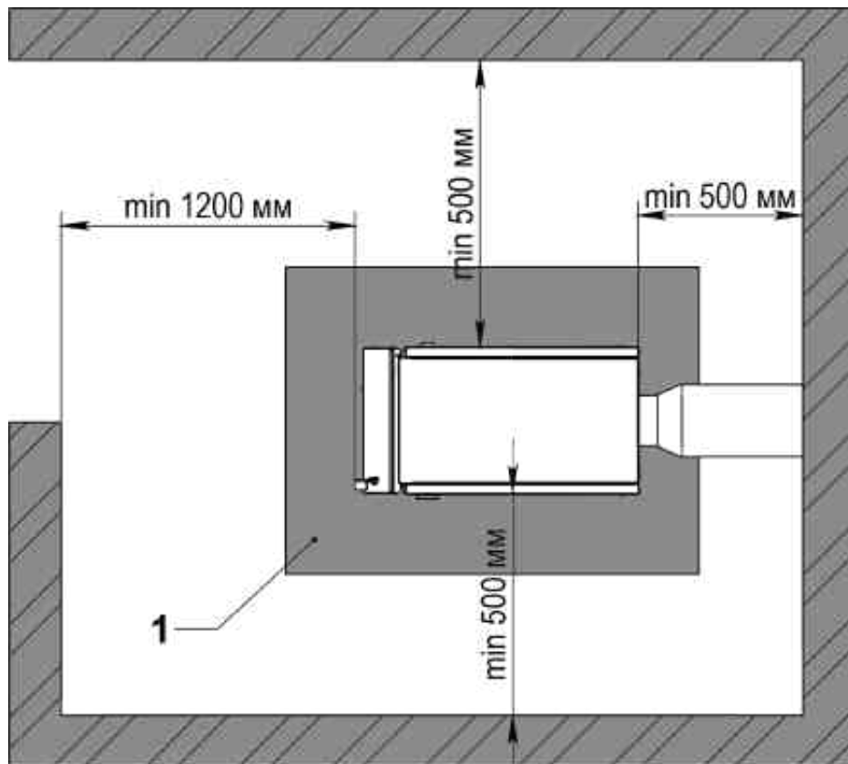
Рис. 4 Установка котла
