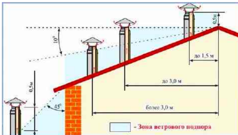
Рис. 11 Высота дымохода
