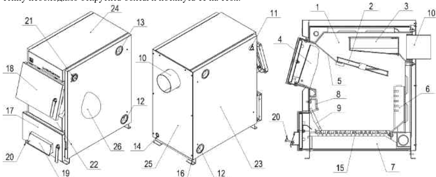
Рис. 1 Устройство котла
