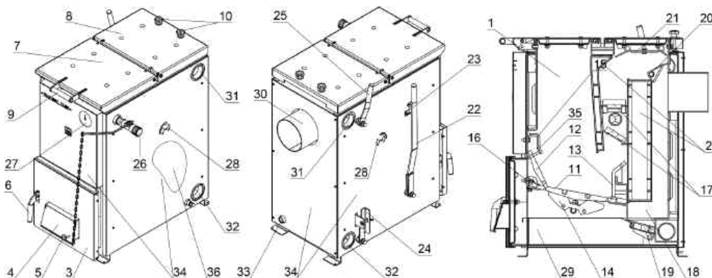
Рис. 1 Устройство котла ZEUS
