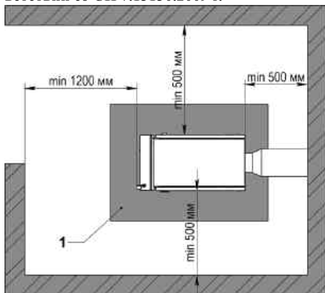
Рис. 3 Установка котла
