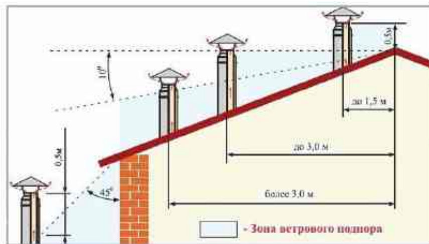
Рис. 7 Высота дымохода.
