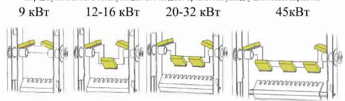
Рис. 8 Схема укладки шамотных кирпичей.
